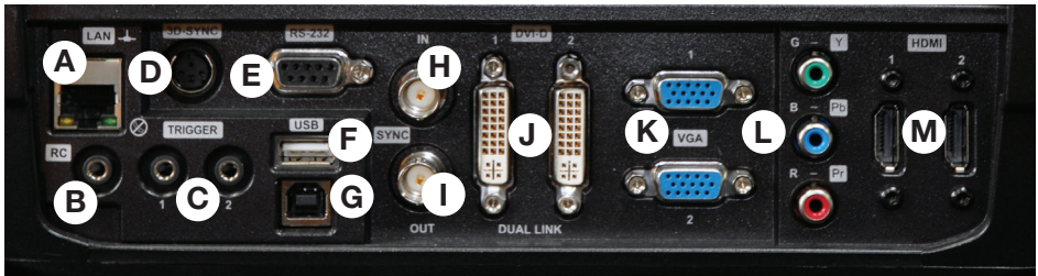
图 4-7. 连接器面板
